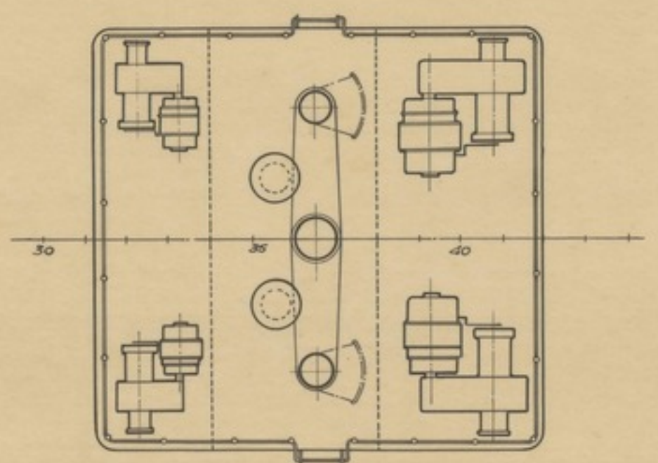
Plataforma de Chigres MASTHOUSE TOP
