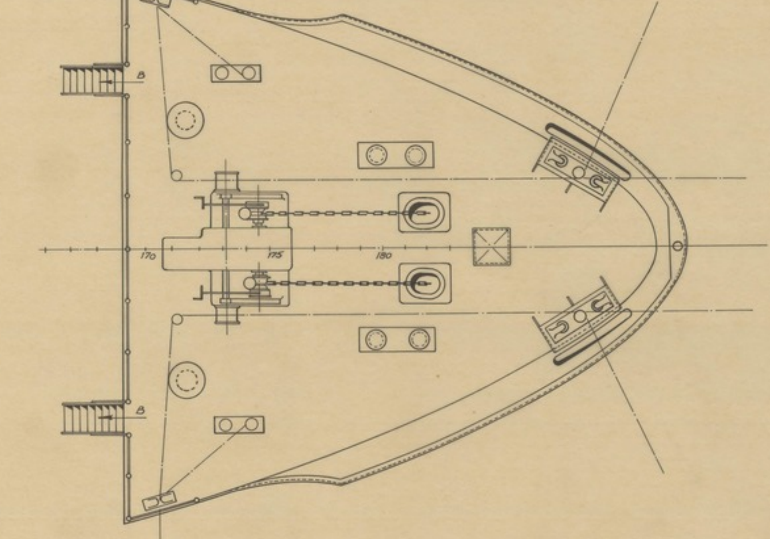
Cubierta Castillo FORECASTLE DECK.
