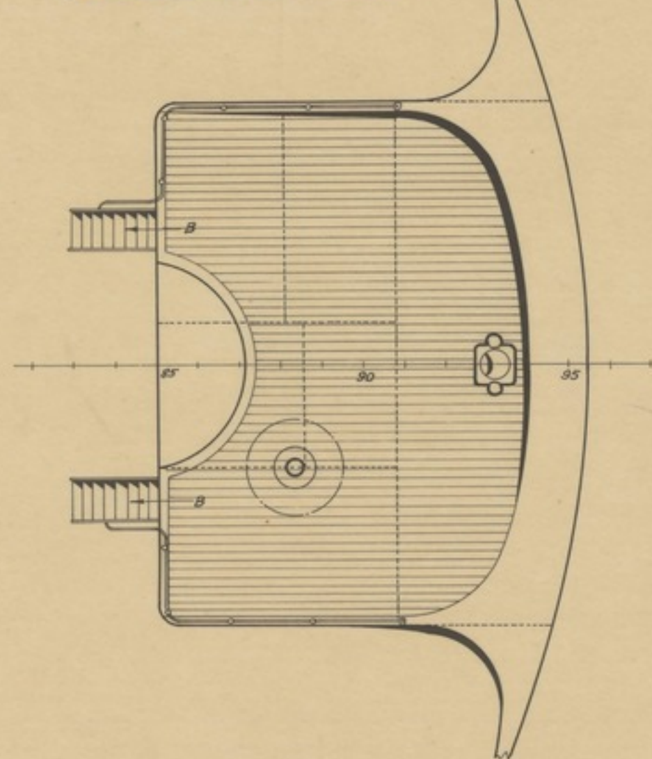
Techo del Puente WHEEL HOUSE TOP.
