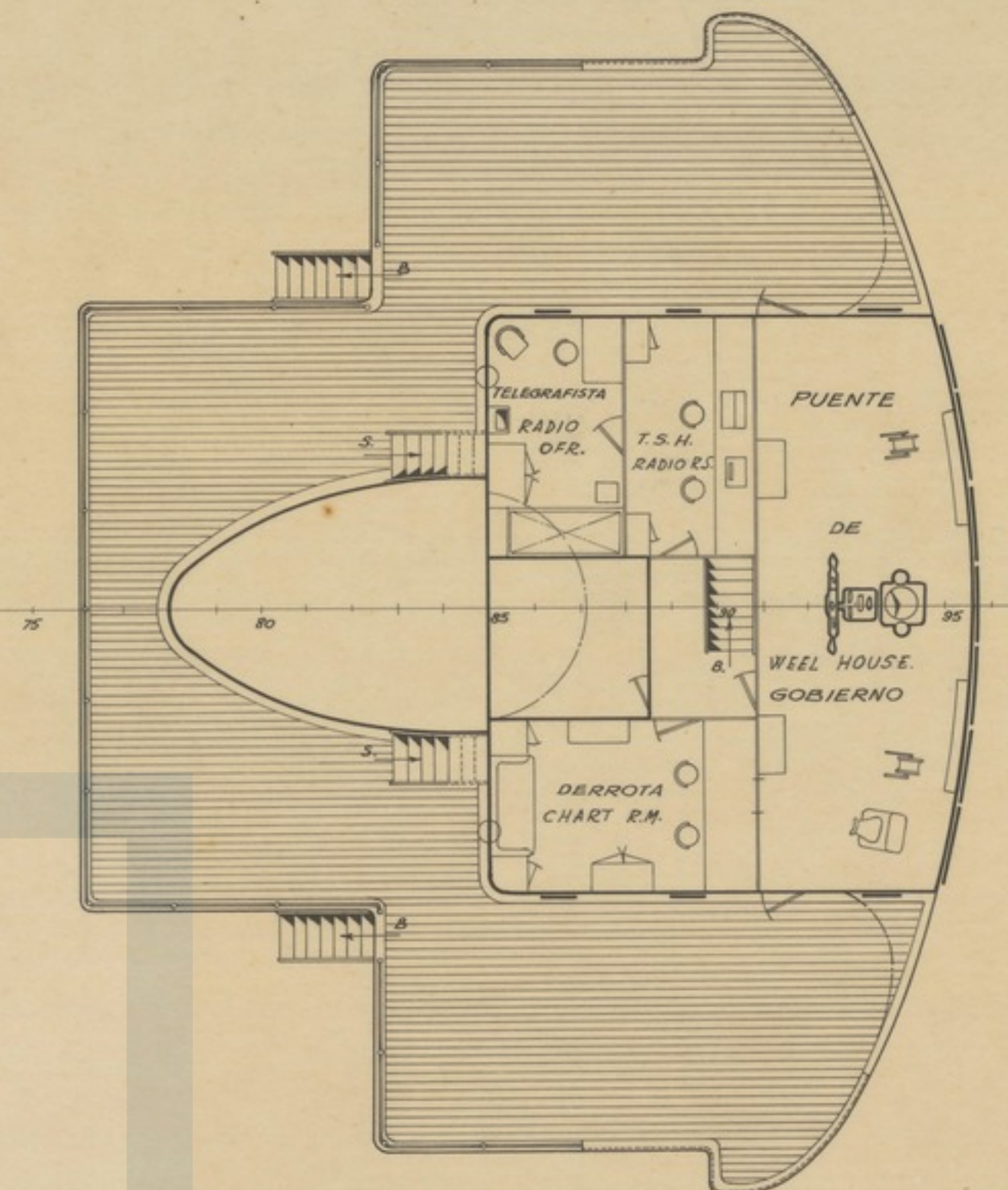
Cubierta de Puente NAVIGATING BRIDGE.
