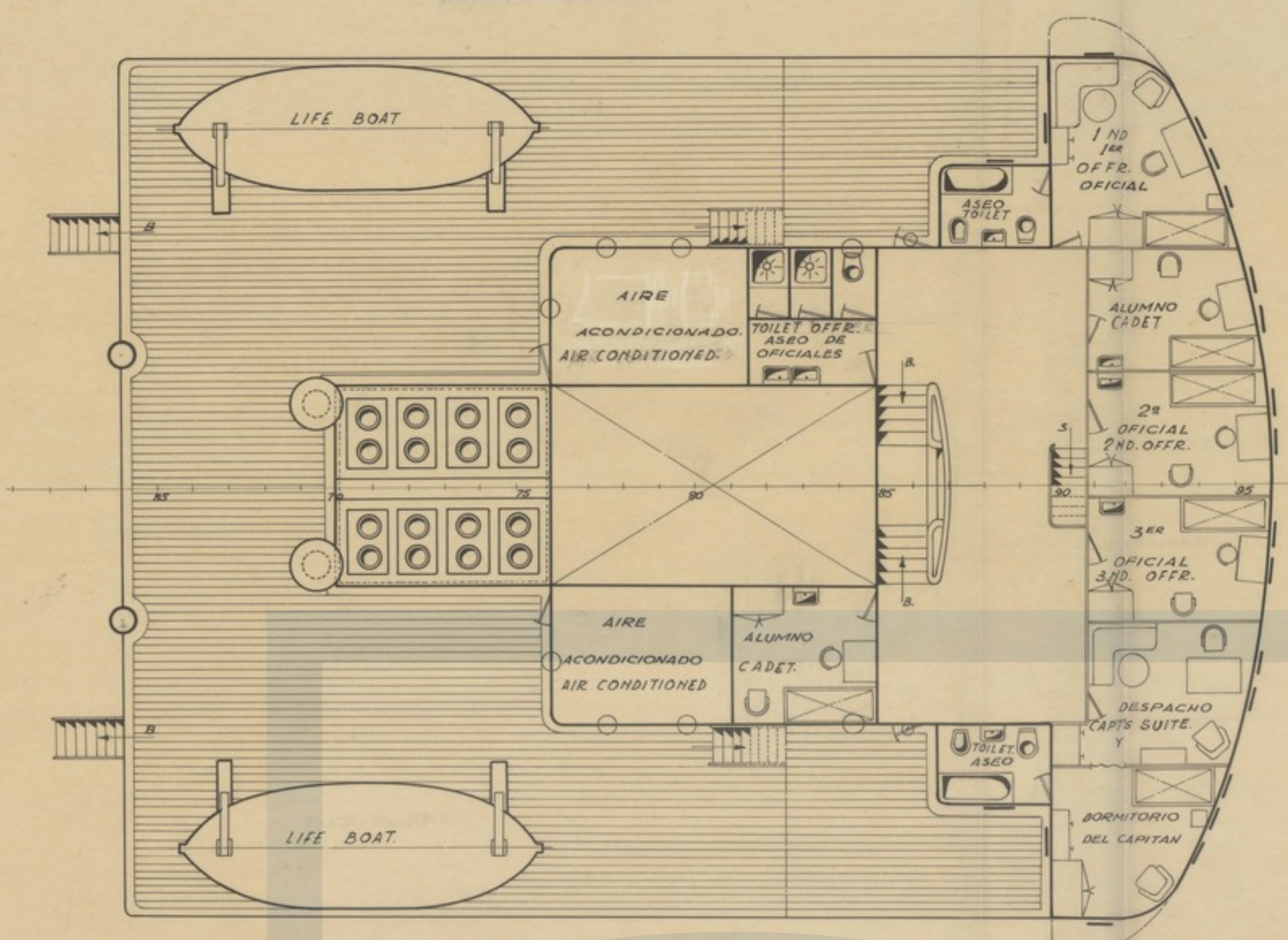
Cubierta Ciudadela BRIDGE DECK.
