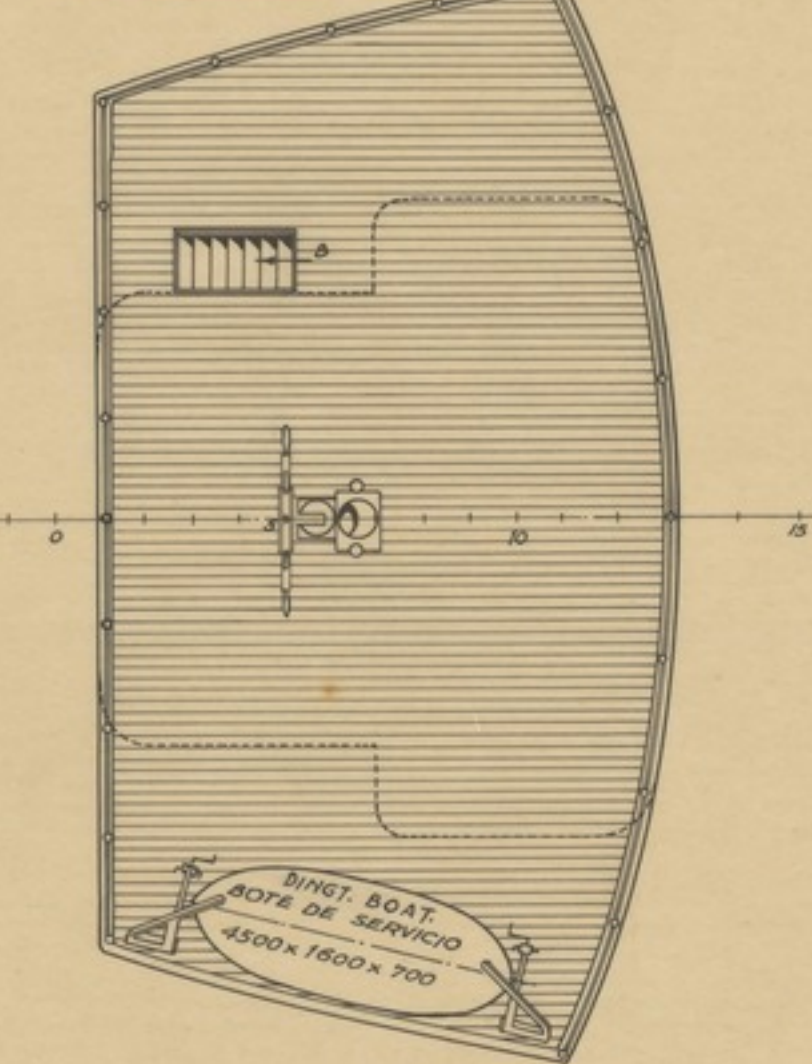
Cubierta Toldilla POOP DECK.
