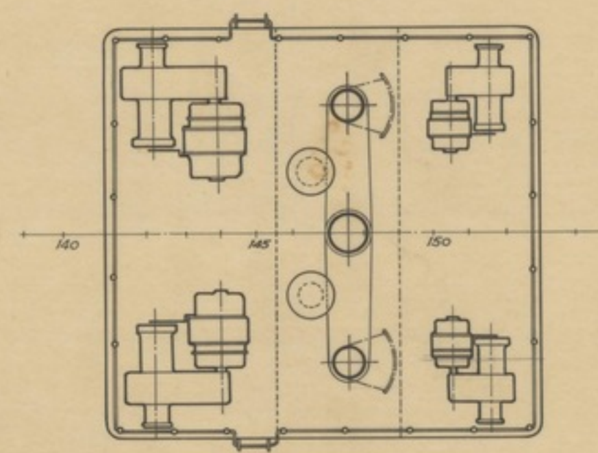
Plataforma de Chigres MASTHOUSE TOP
