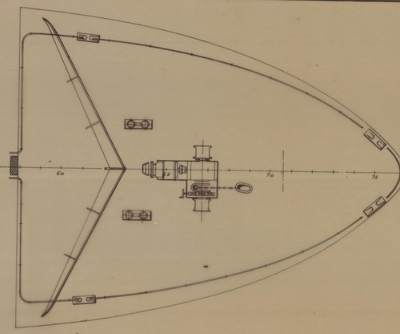
Cubierta Principal
