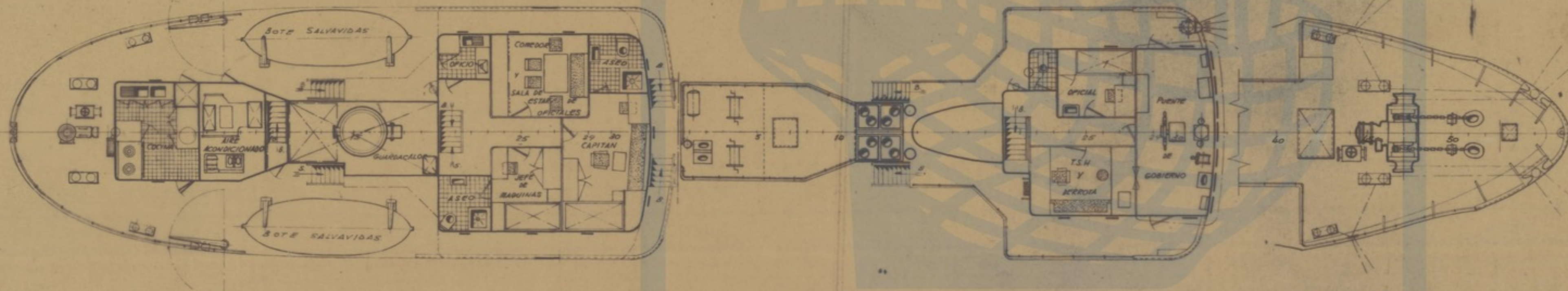
Cubierta Principal
