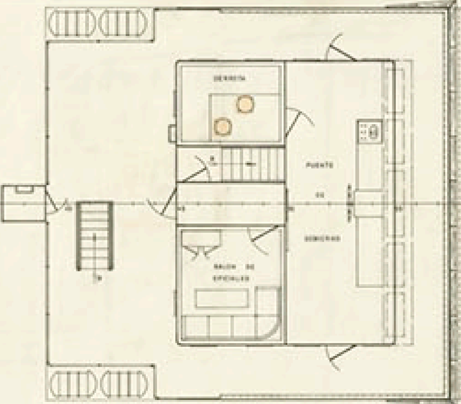
CUB PUENTE
