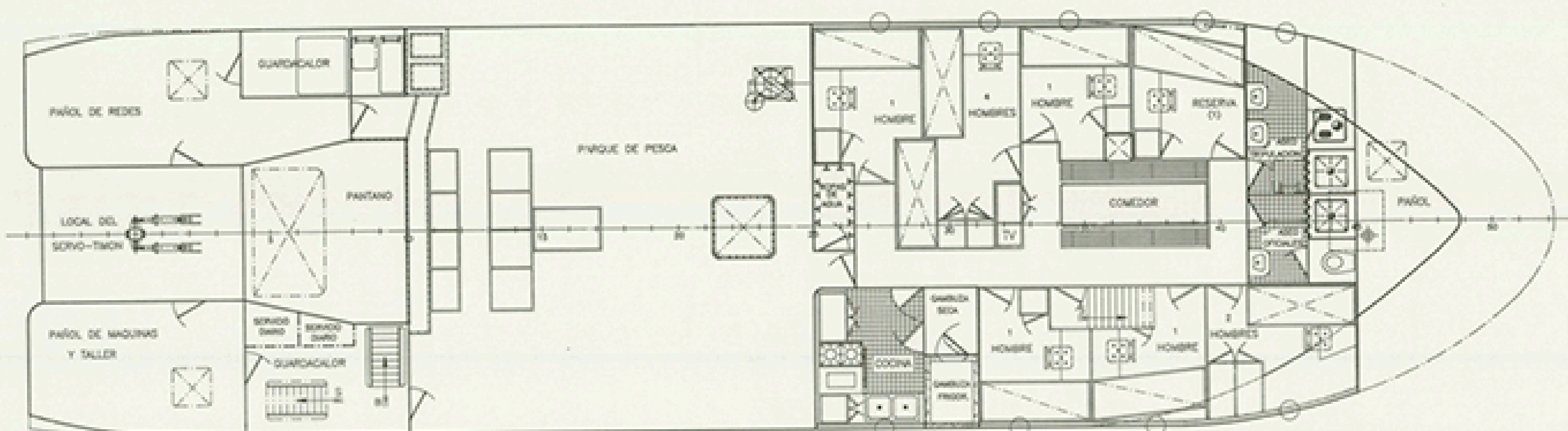
CUBIERTA PRINCIPAL
