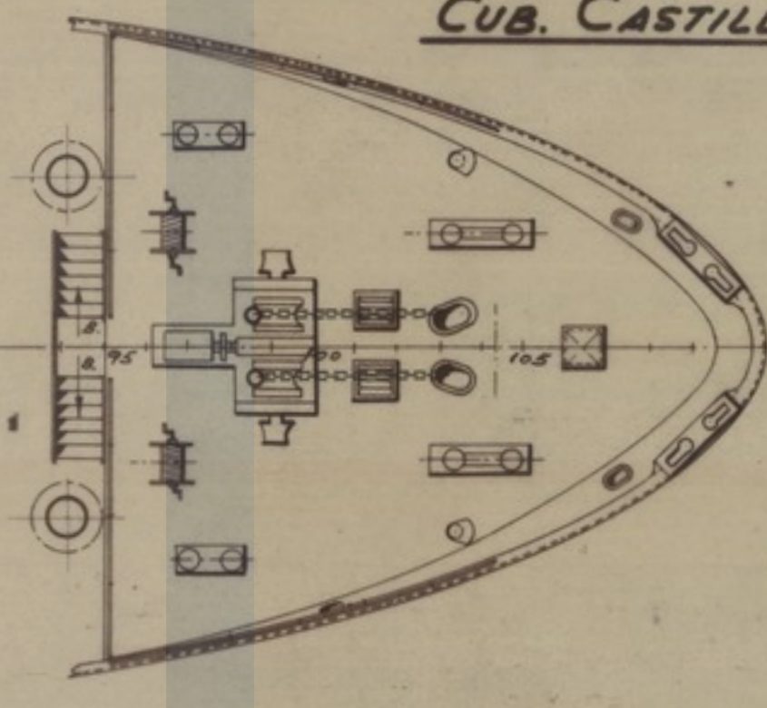
CUB. CASTILLO.
