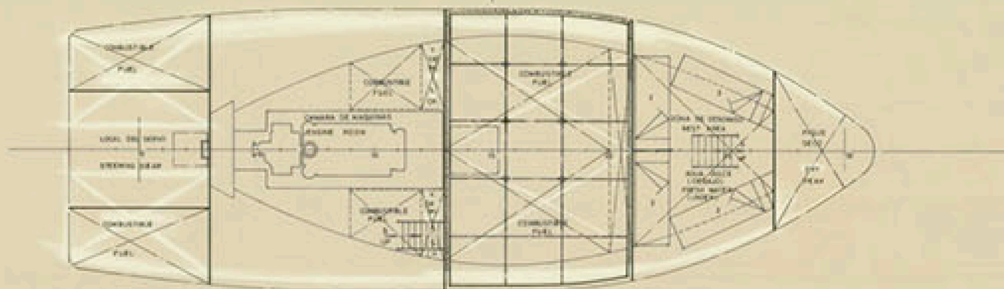
DOBLE FONDO DOUBLE BOTTOM
