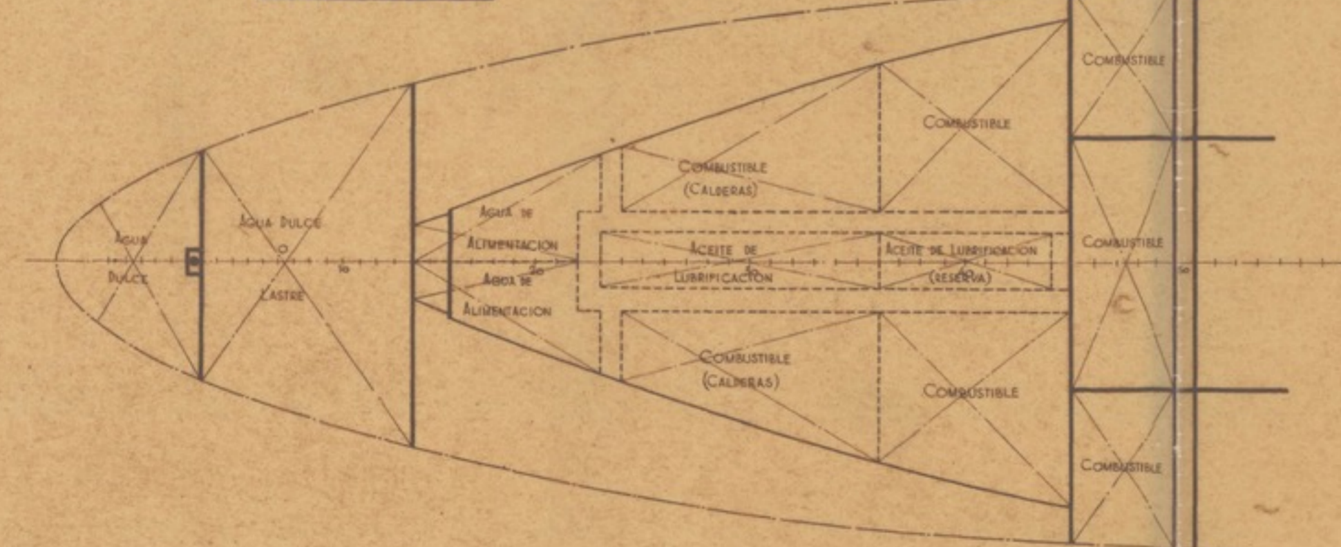
DOBLE FONDO
