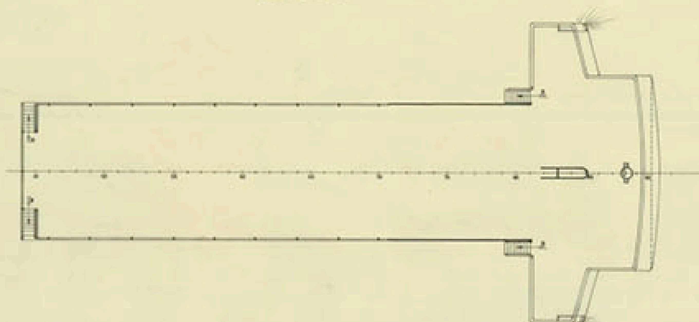
CUB. PUENTE (Deck Plan)
