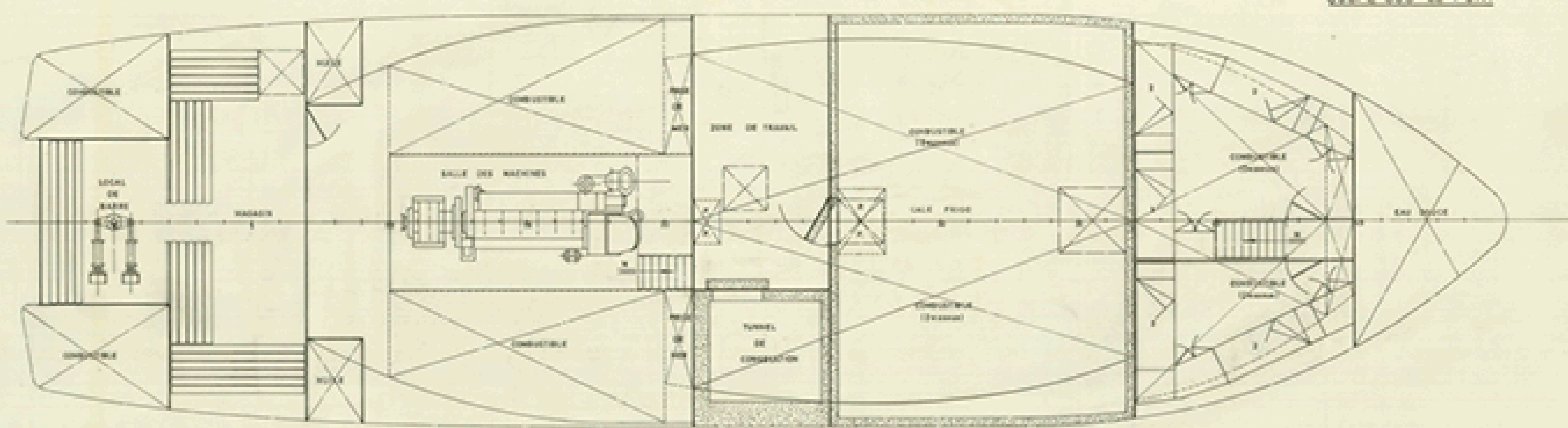
COUPE SUS LE PONT
