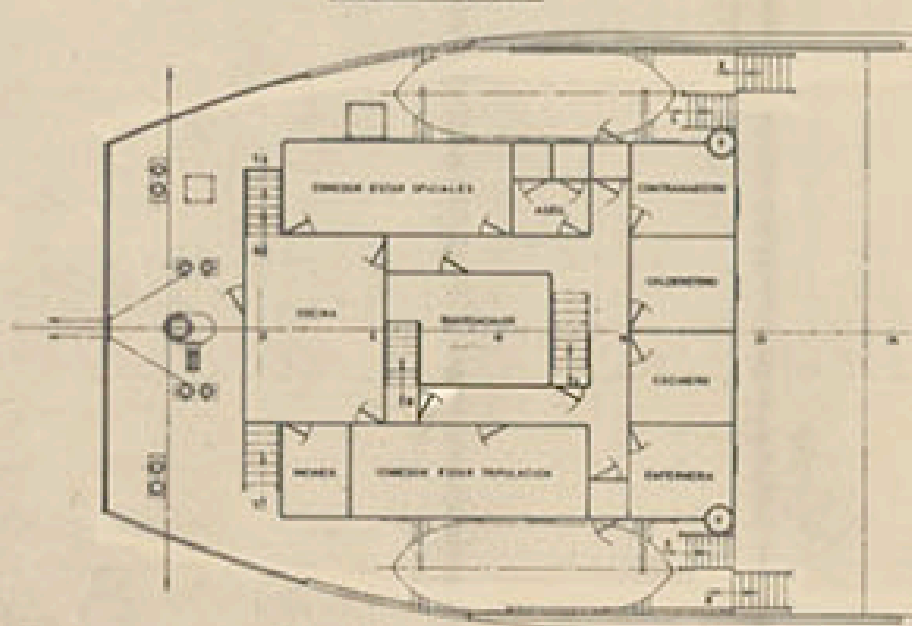
CUBIERTA TOPELLA
