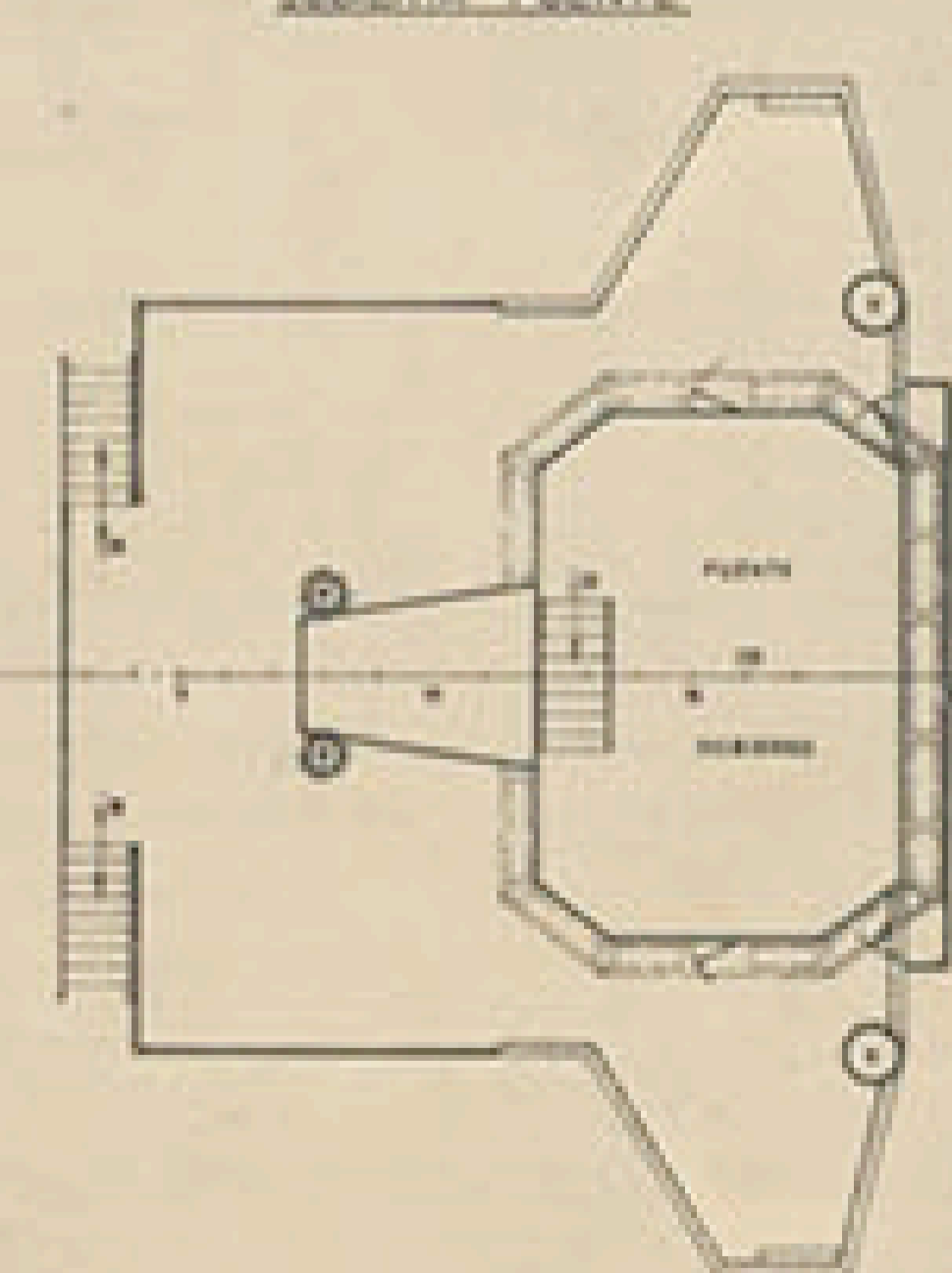
CUBIERTA PUENTE
