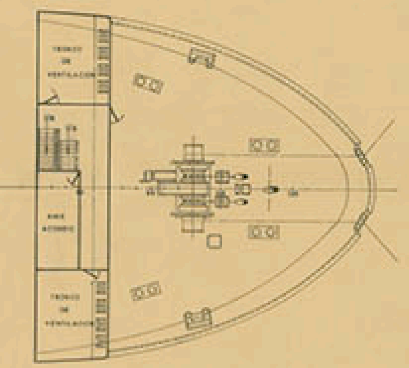
CUBIERTA CASTILLO
