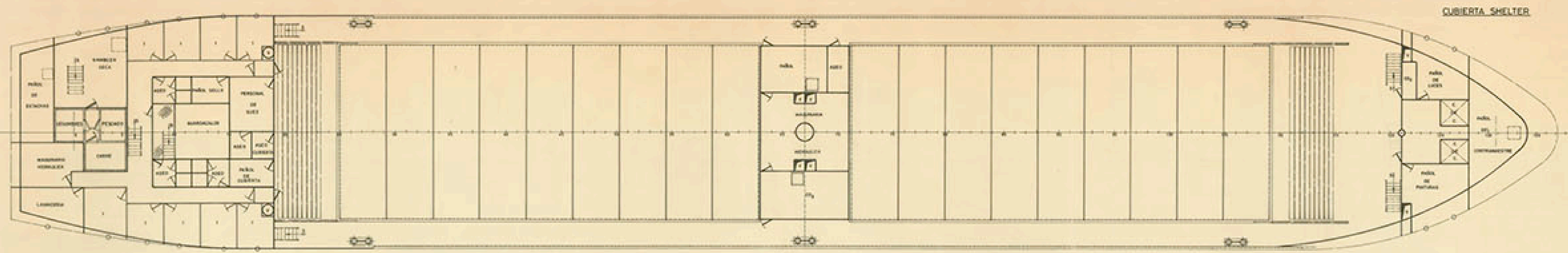
CUBIERTA SHELTER
