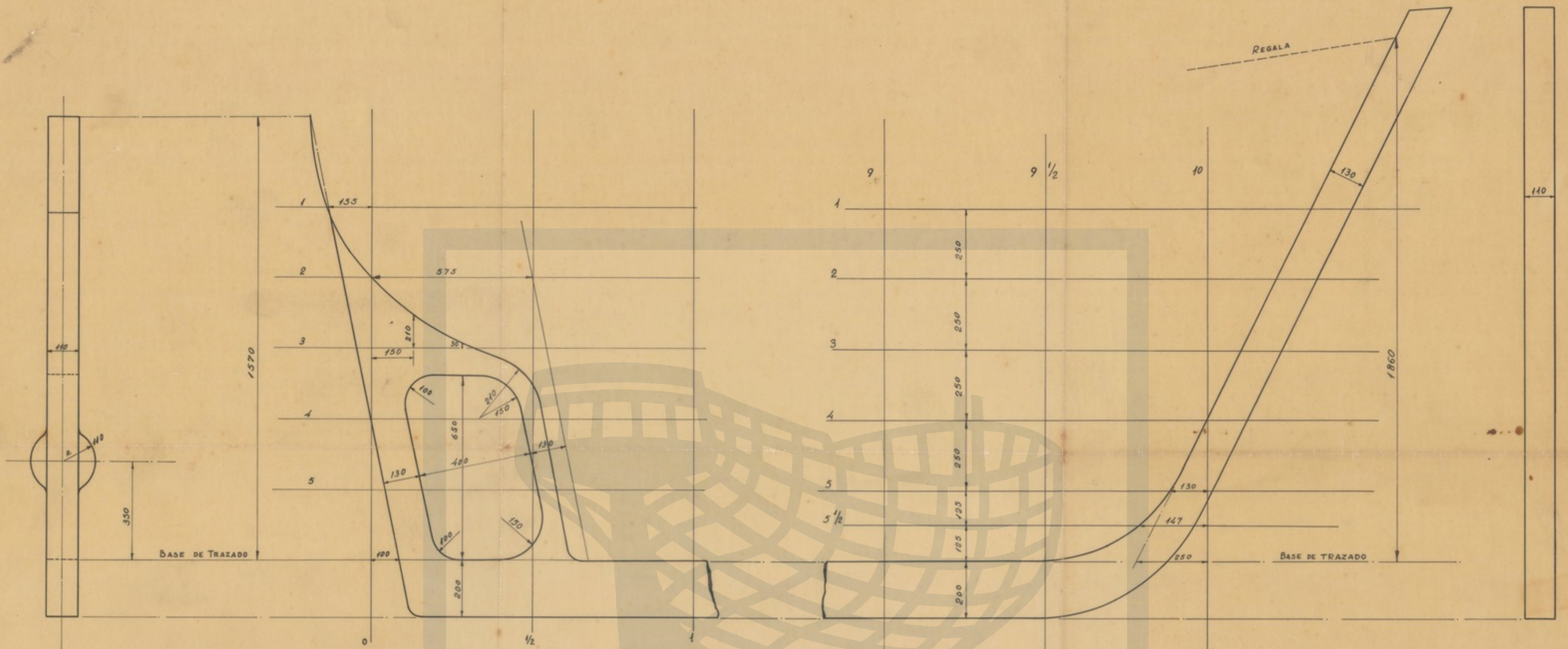
TRAZADO DEL CODASTE
