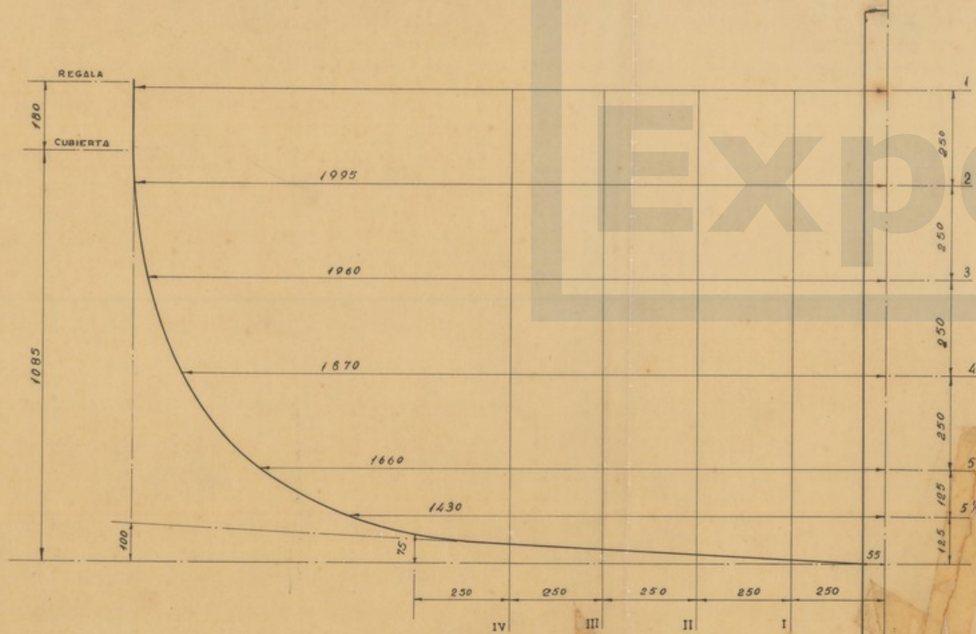
TRAZADO DE LA SECCIÓN 5
