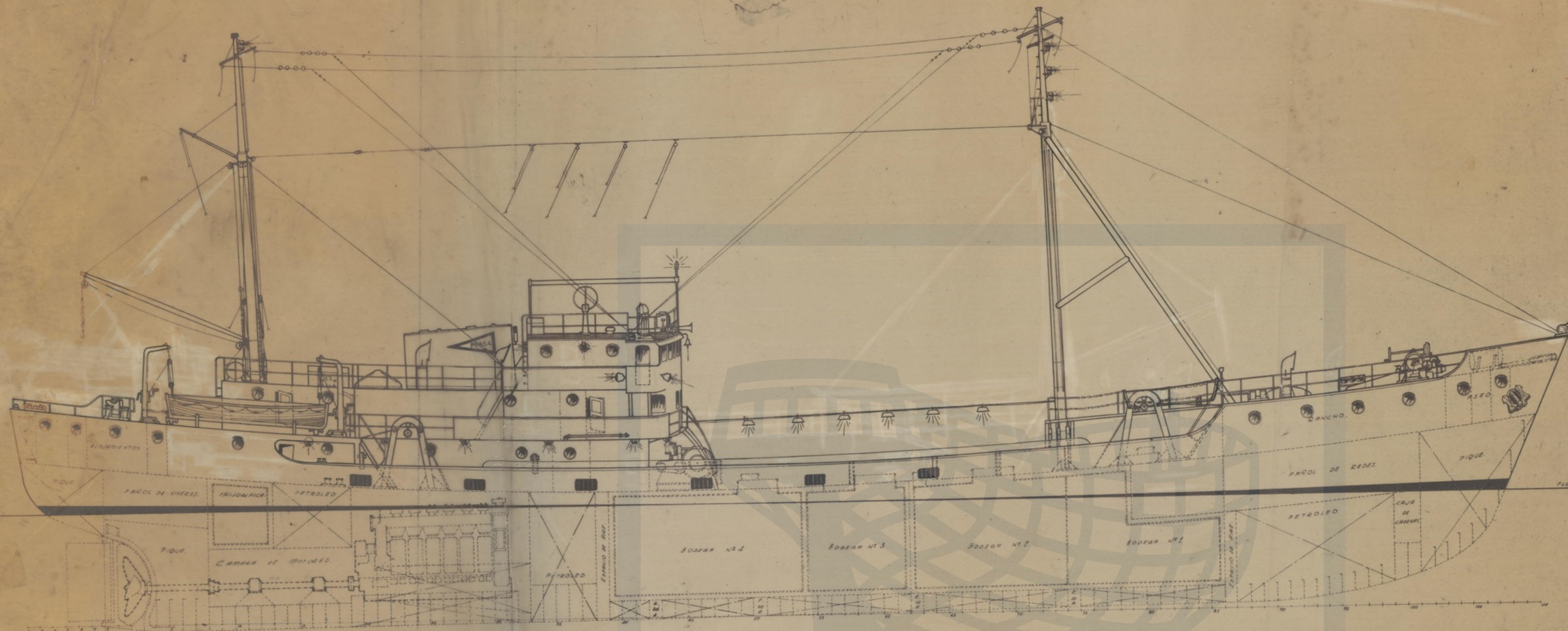
PERFIL.
