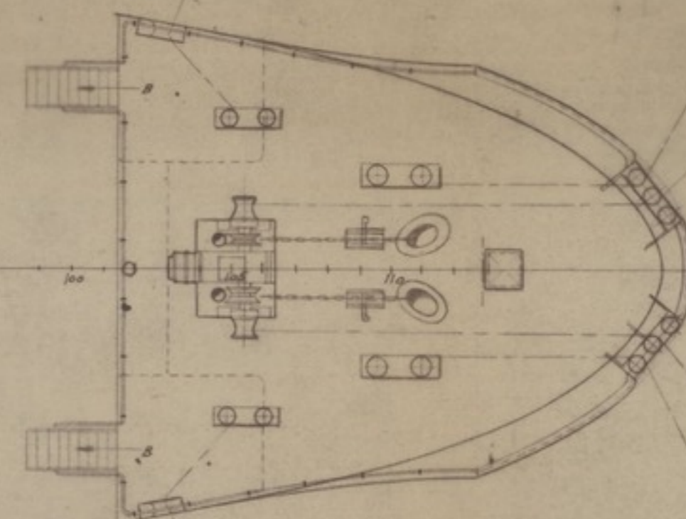
Cubierta Shelter
