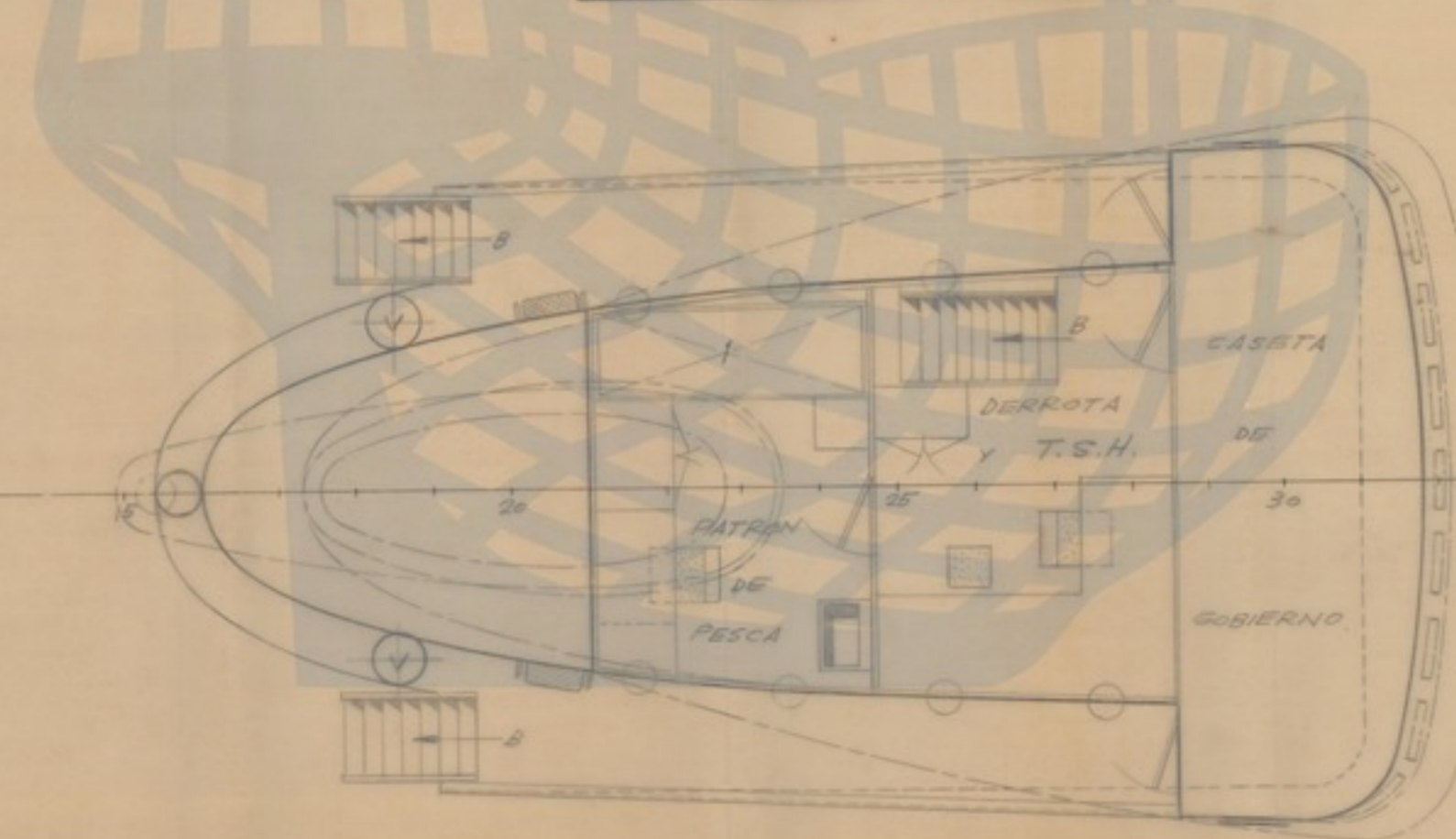
Cubierta Puente
