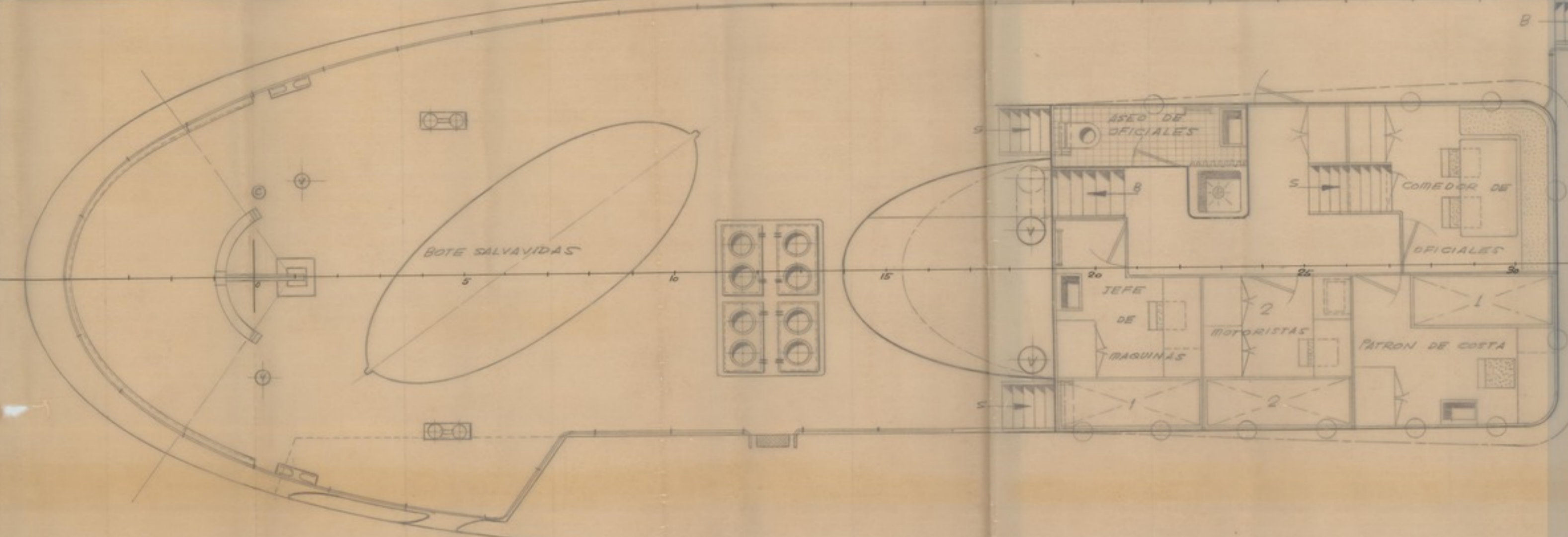
Cubierta Toldilla
