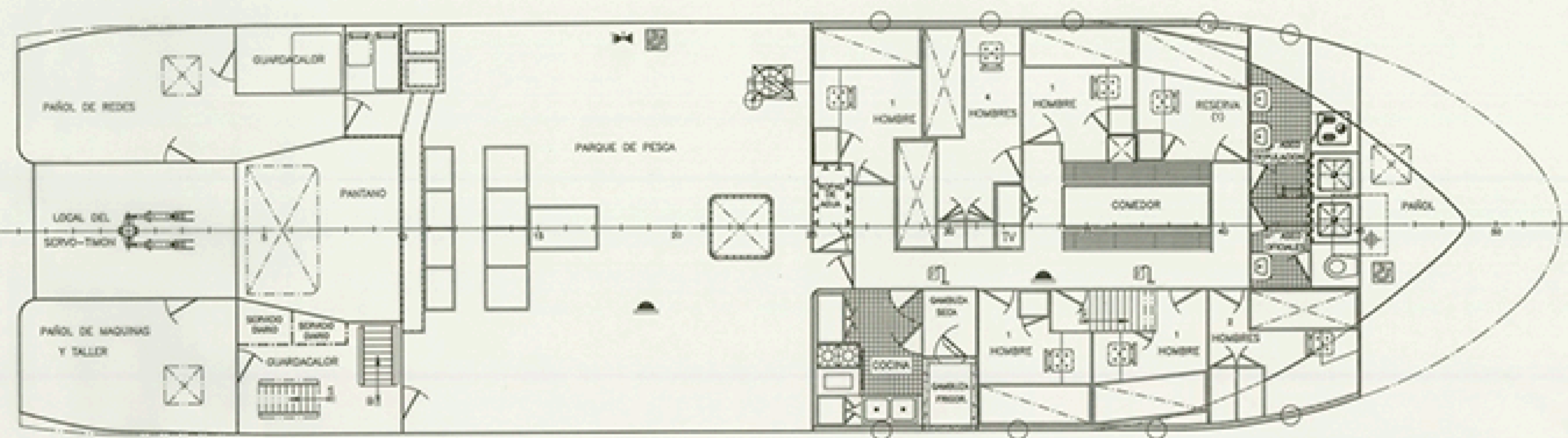
CUBIERTA PRINCIPAL
