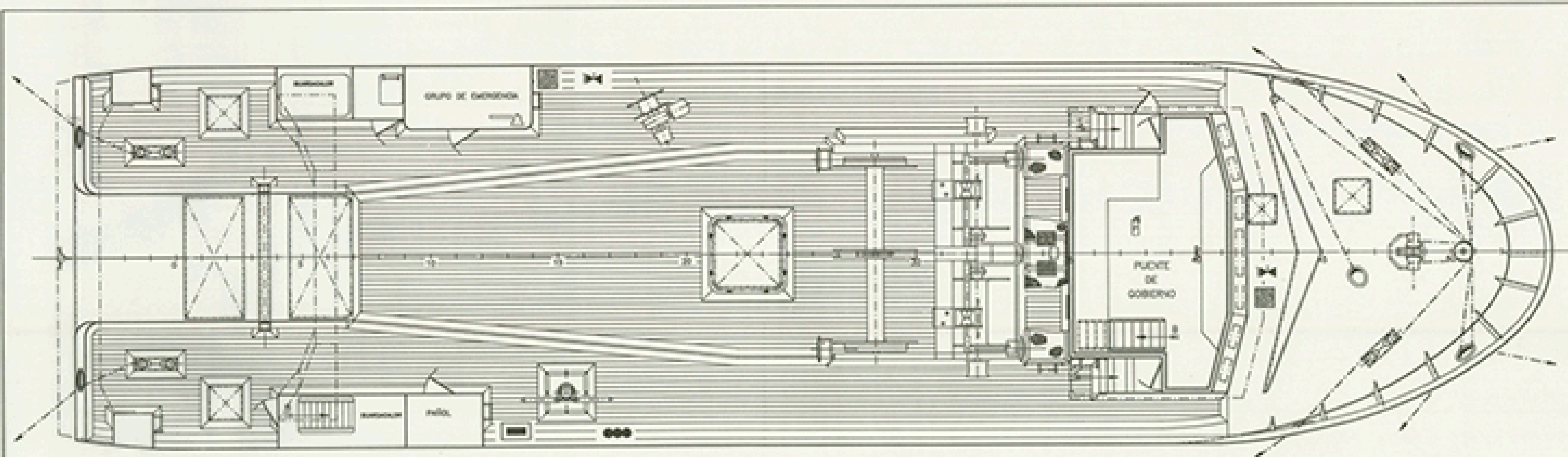
CUBIERTA SUPERIOR
