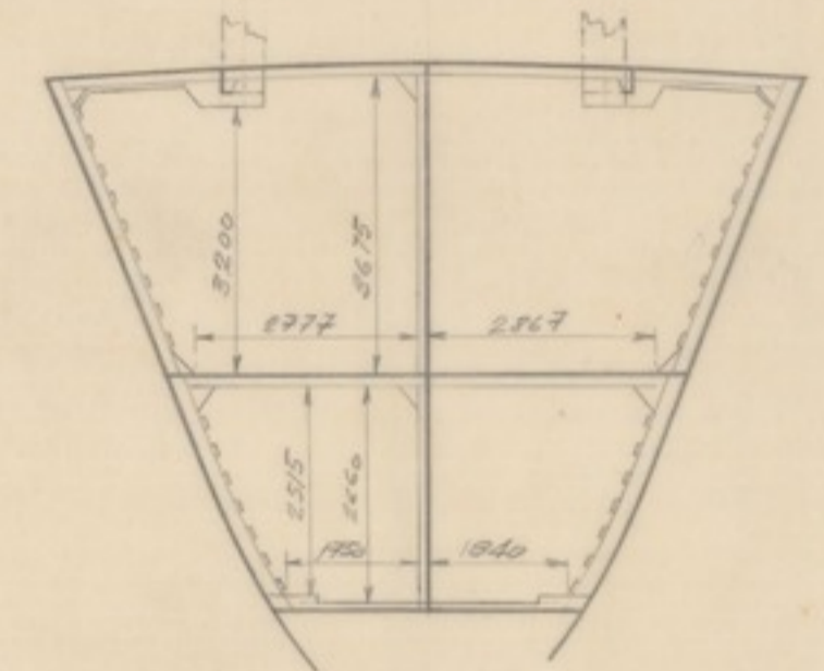
SECCION POR LA C M 7/2 (Mirando a popa)
