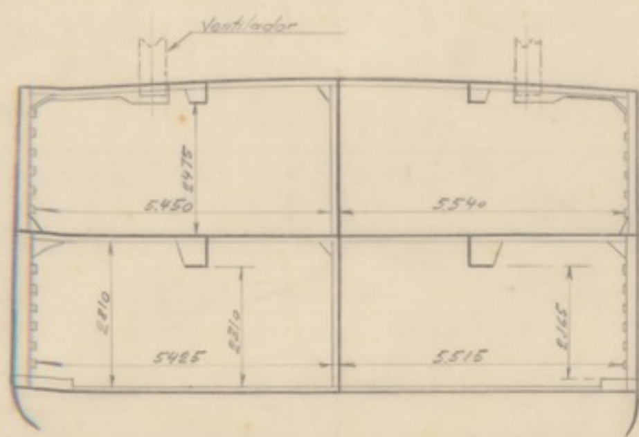
SECCION POR LA C M 5/2 (Mirando a popa)
