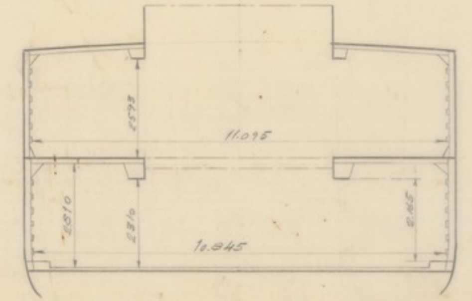
SECCION POR LA C M 6/2 (Mirando a popa)
