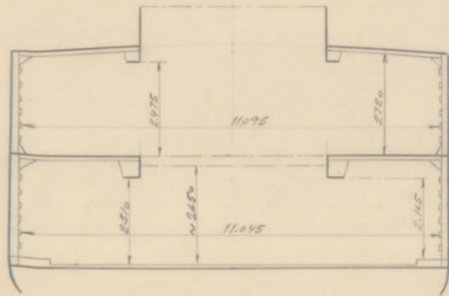
SECCION POR LA C M 5/1 (Mirando a popa)
