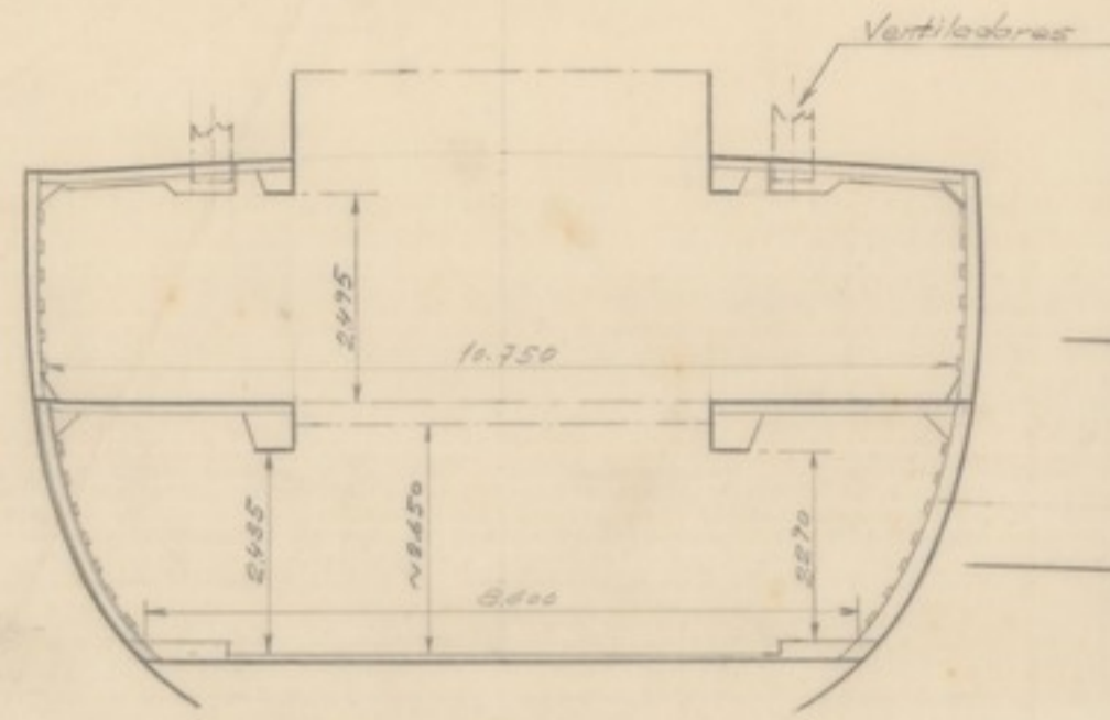
SECCION POR LA C M 3/1 (Mirando a popa)
