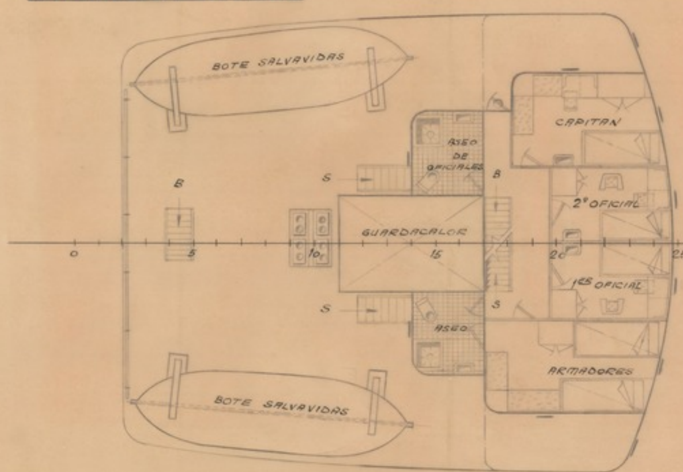
CUBIERTA BOTES
