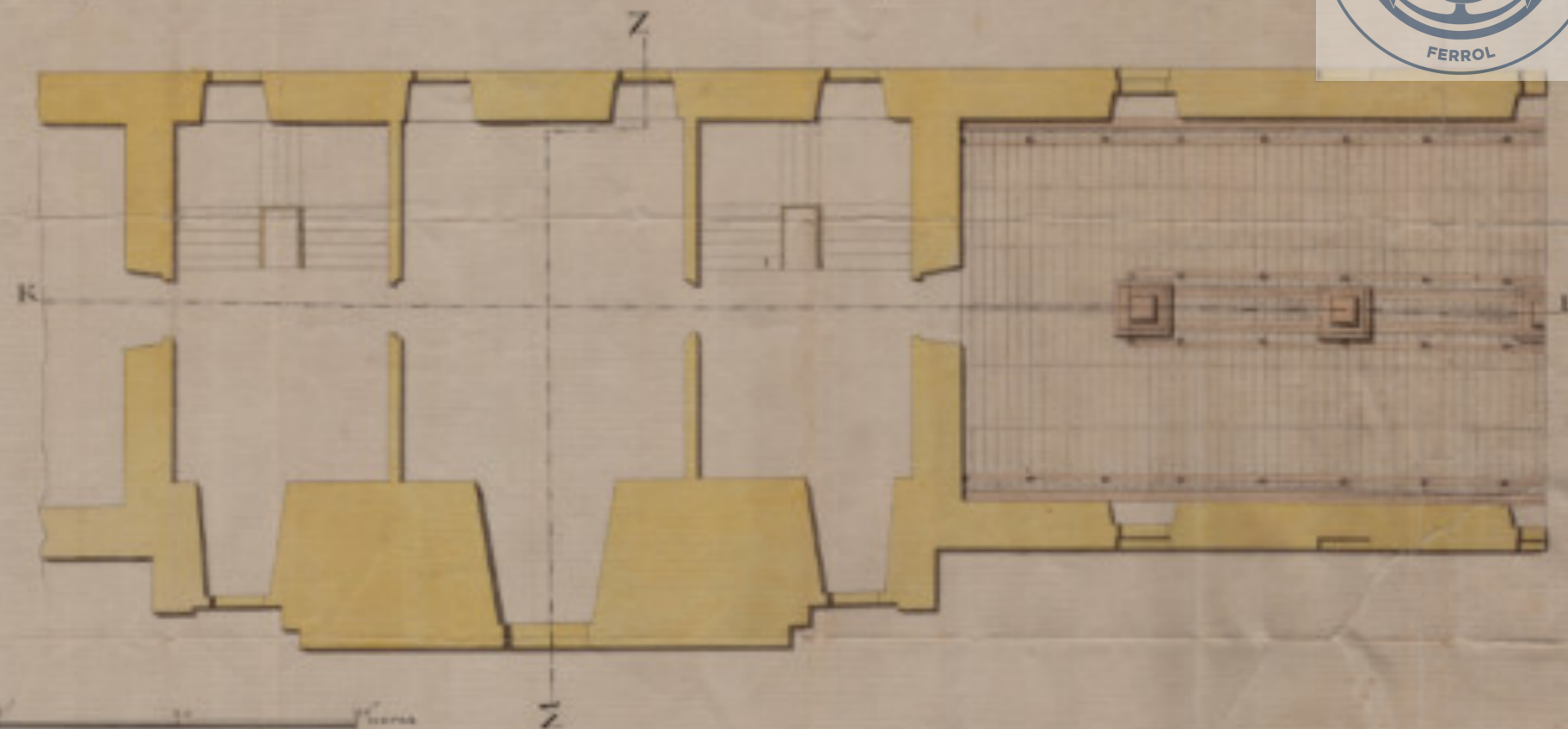
PLANO de encima dha Escalera y Almacenes en q demuestrá una porcion de la Sala de Armas con su escalera y aleros de las paredes como tambien el Armazon para Colocar las Armas
